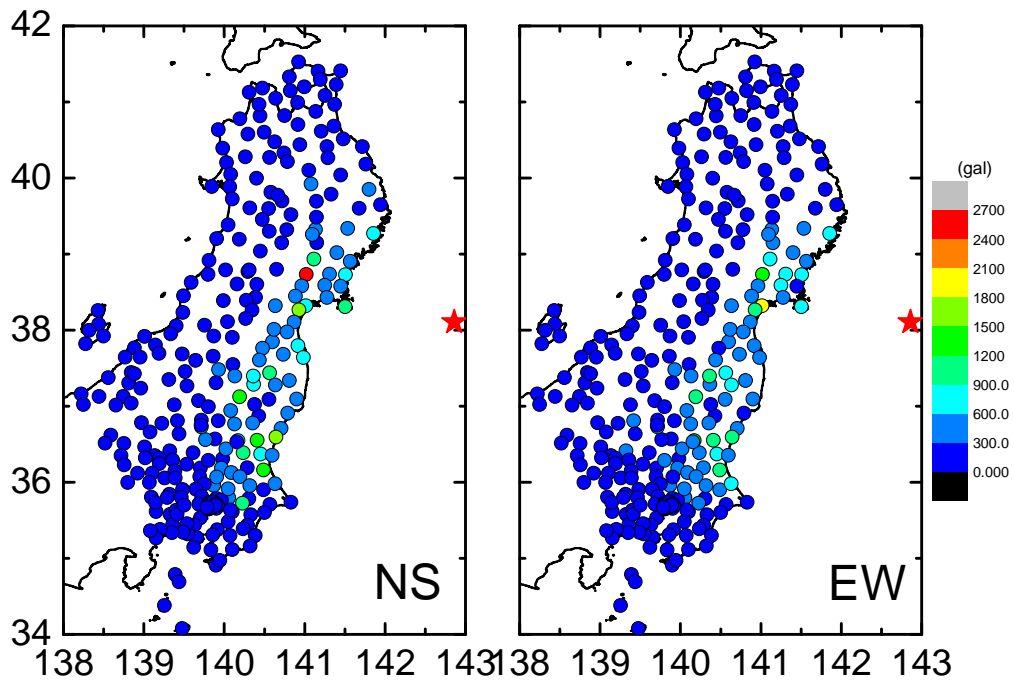
最大加速度分布 (左 : NS 方向, 右 : EW 方向)
