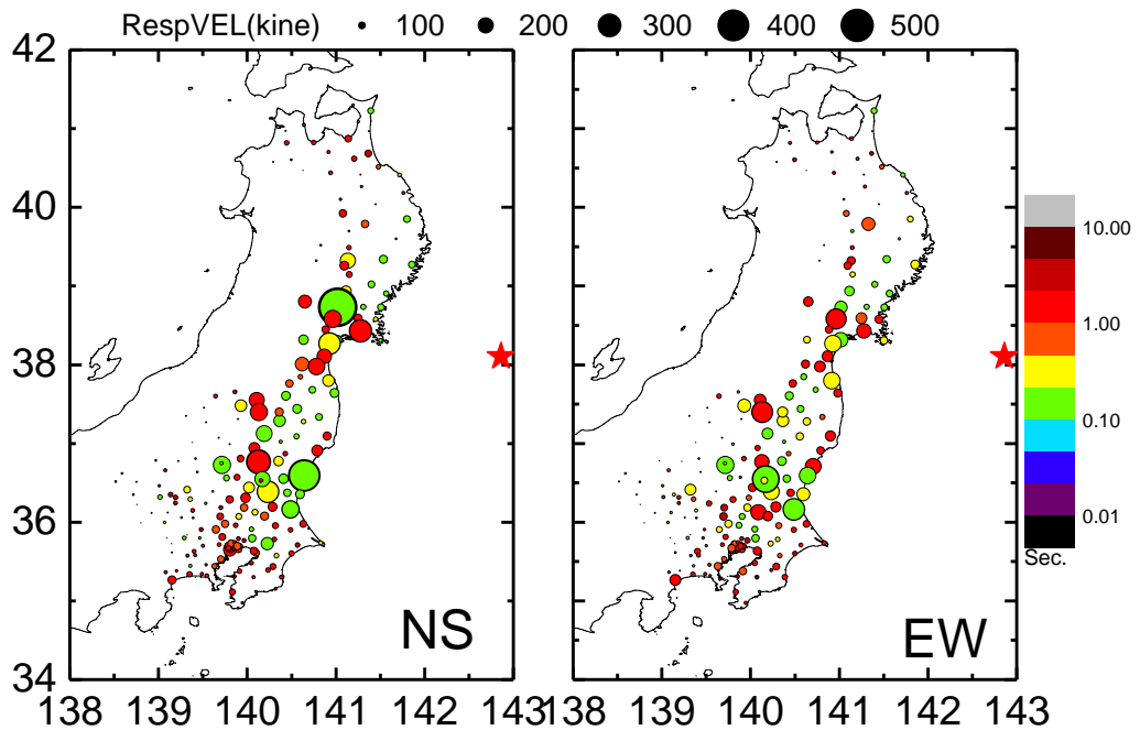
速度応答スペクトルのピーク値分布（左：NS方向，右EW方向）
