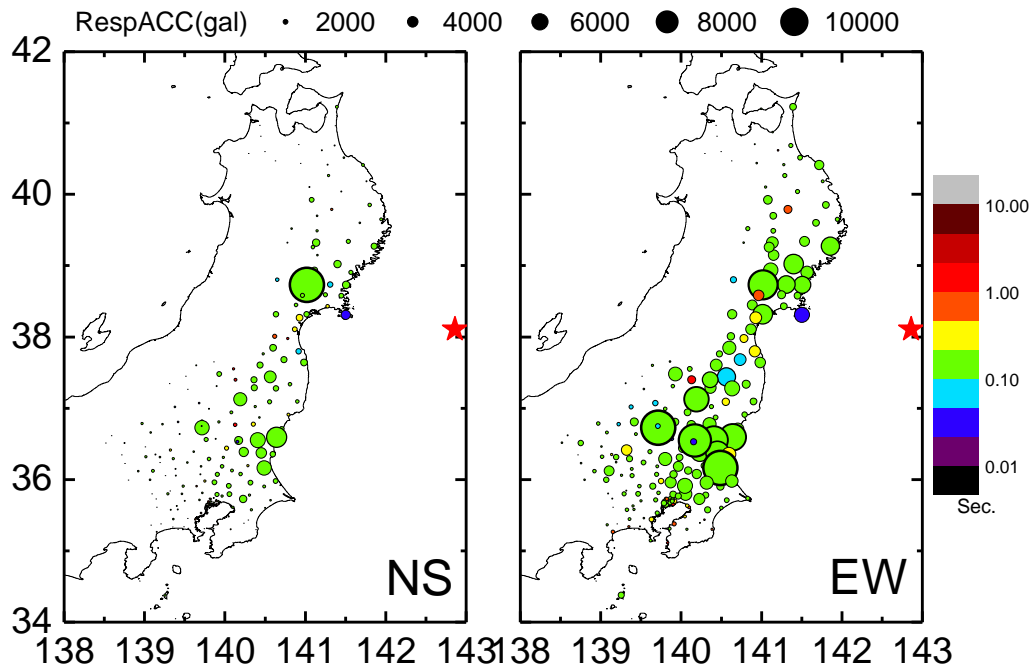
加速度応答スペクトルのピーク値分布（左：NS方向，右EW方向）
