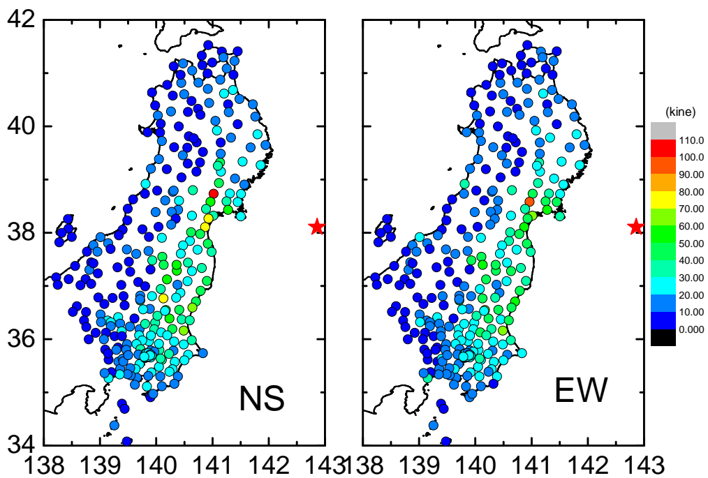
最大速度分布 (左 : NS 方向, 右 EW 方向)
